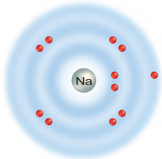
ذرة صوديوم
